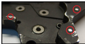
Obr. 6 - při tlusté kabeláži zbruste výstupky na mechaboxu
