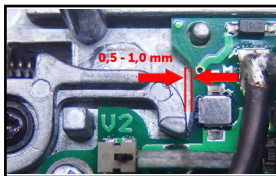
Obr. 2 - mezera mezi přerušovačem a mikrosplínáčem na procesorovce
